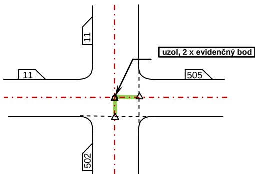
Obrázok 4a Detail križovatky, kolmé napojenie, priesečné
